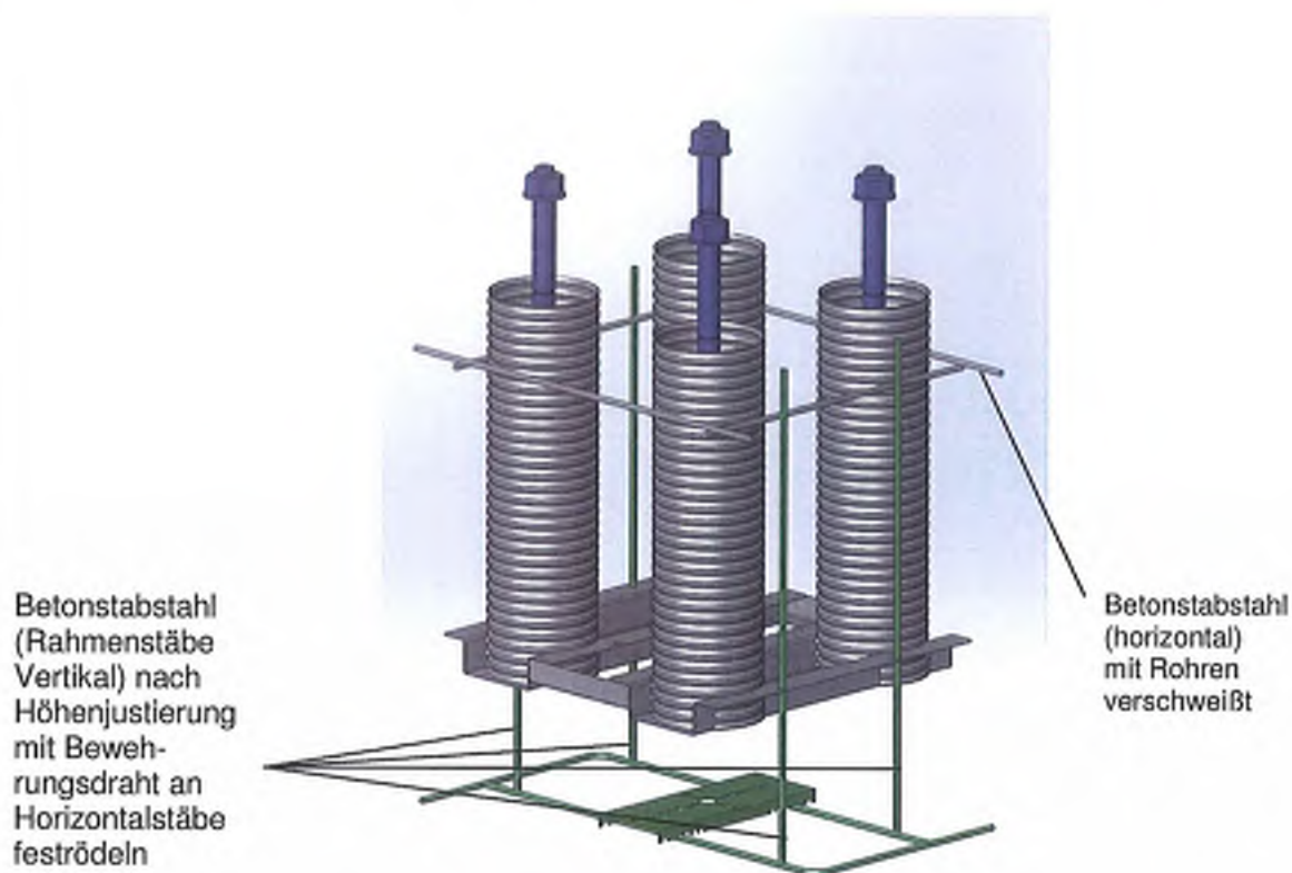
Nachjustierbare einbaufertige Haltevorrichtung (Rahmen)
